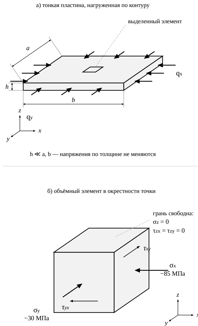
Рис. 1 — тонкая пластина, нагруженная по контуру (а), и выделенный из неё объёмный элемент (б): грани с нормалью z свободны от напряжений.
