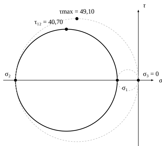
Рис. 8 — три круга Мора, по одному на каждую пару главных напряжений. Сплошной — пара \sigma_1, \sigma_2 (он же основной круг п. 9), радиус 40,70 МПа. Наибольший радиус у пары \sigma_2, \sigma_3 — это и есть \tau_{\max} = 49,10 МПа.
