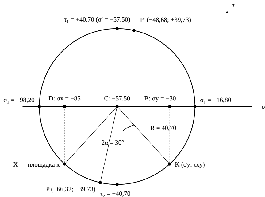
Рис. 7 — круг Мора. Построение: D и B — исходные \sigma_x и \sigma_y на оси; C — центр; BK = \tau_{xy} отложено от B вниз; R = CK. С круга снимаются \sigma_1 и \sigma_2 (пересечения с осью), \tau_1 и \tau_2 (верх и низ), точка P — площадка под \alpha = 15^\circ , P' — перпендикулярная ей. Все шесть величин совпали с аналитическим расчётом.
