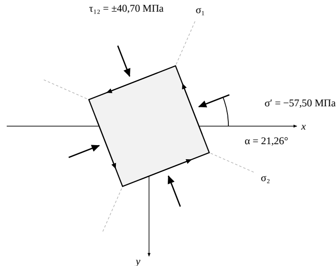
Рис. 4 — площадки с \tau_{12} = \pm 40,70 МПа в плоскости пластины. Элемент повернут на 45^\circ от главных направлений: \alpha = 66,26^\circ - 45^\circ = 21,26^\circ . Штриховыми показаны главные направления, на всех четырёх гранях \sigma' = -57,50 МПа.
