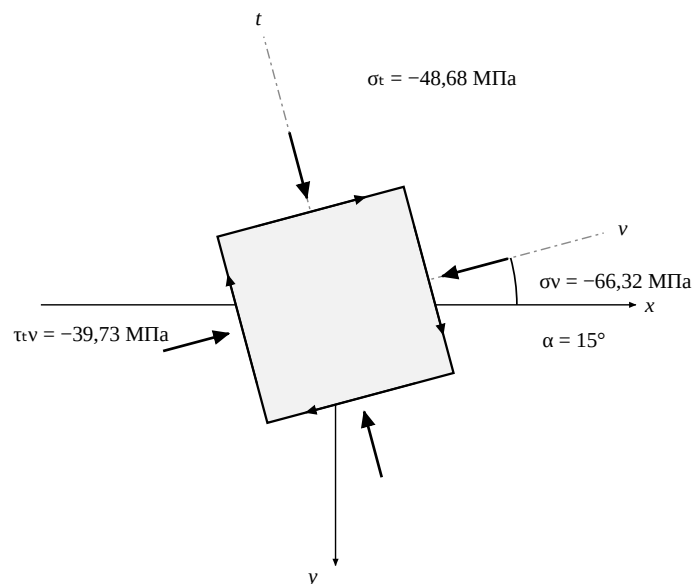
Рис. 5 — напряжения на площадках, повёрнутых на \alpha = 15^\circ . Оба нормальных напряжения сжимающие, стрелки направлены к граням; касательные образуют уравновешенную пару.
