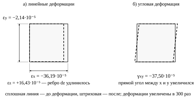
Рис. 6 — деформация элемента. Слева линейные деформации: ребро dx укоротилось заметно, dy почти не изменилось, dz удлинилось (вдоль свободной от нагрузки оси z ). Справа угловая деформация: прямой угол между осями x и y увеличился, потому что \gamma_{xy} отрицательна.
